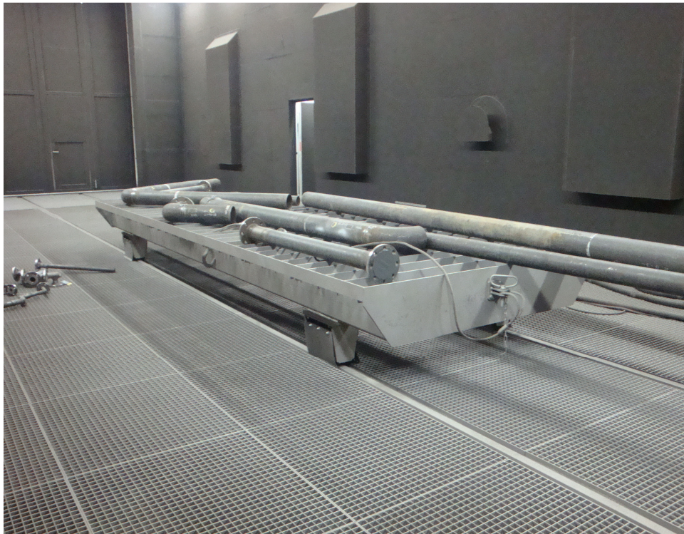
Strahlhalle Mehrwegstrahlmittel 22,00 m lang, 5,00 m breit, max. 5,00 m hoch
